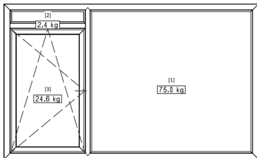
Nieuwe situatie kozijnen en draai-kiepraam (of in spiegelbeeld)
